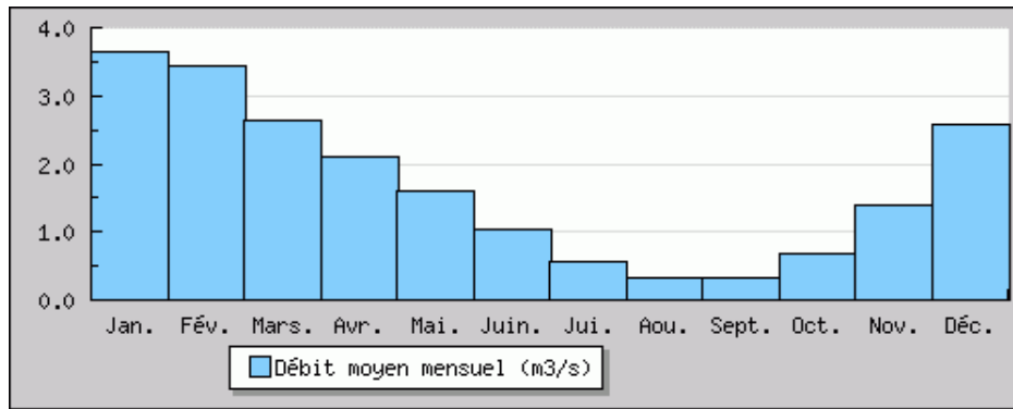
Figure 9: Débit moyen mensuel de la Claie à Saint-Jean-Brevelay en m3/s (Source: Banque Hydro)
