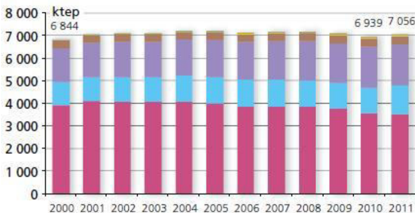
Figure 65: Evolution de la consommation finale d'énergie en Bretagne
