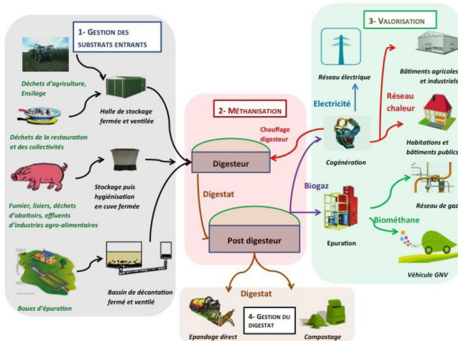
Figure 88 : Principe de fonctionnement d'une unité de méthanisation (Source: ATEE Club Biogaz)
