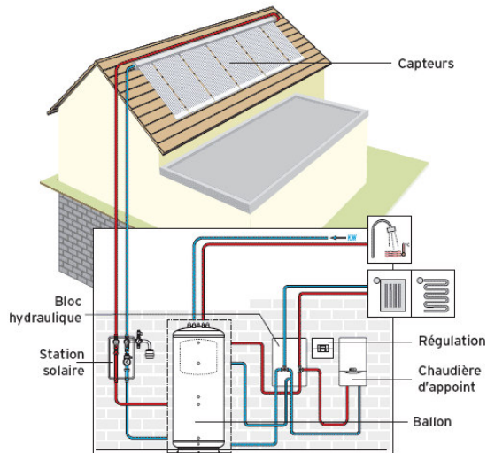
Figure 80 : Principe de fonctionnement d'une installation solaire thermique
